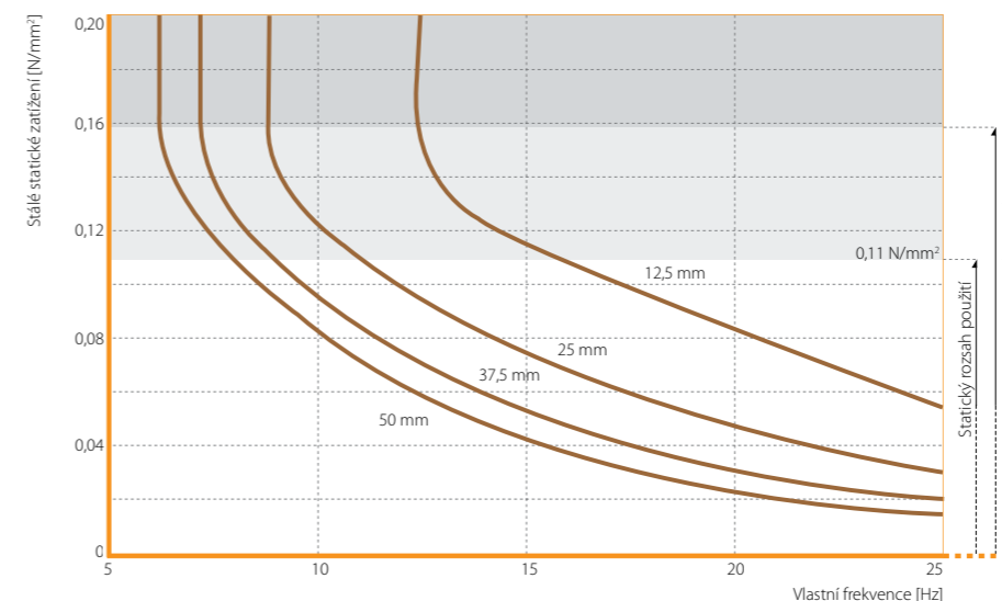
Obr. 3: Vlastní kmitočty volného jednoduňového systému (anglicky „SDOF system“) složený z pevné hmoty a pružné podložky ze SYLOMER® SR 110 uloženého na tuhém podloží
